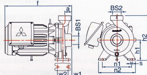
WCM-1505S / WCM-1505T / WCM-2205S / WCM-2205T
