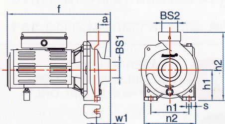
WCM-375S / WCM-755S / WCM-755SH / WCM-1105S
